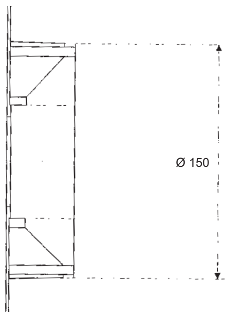
Coupe A-A
